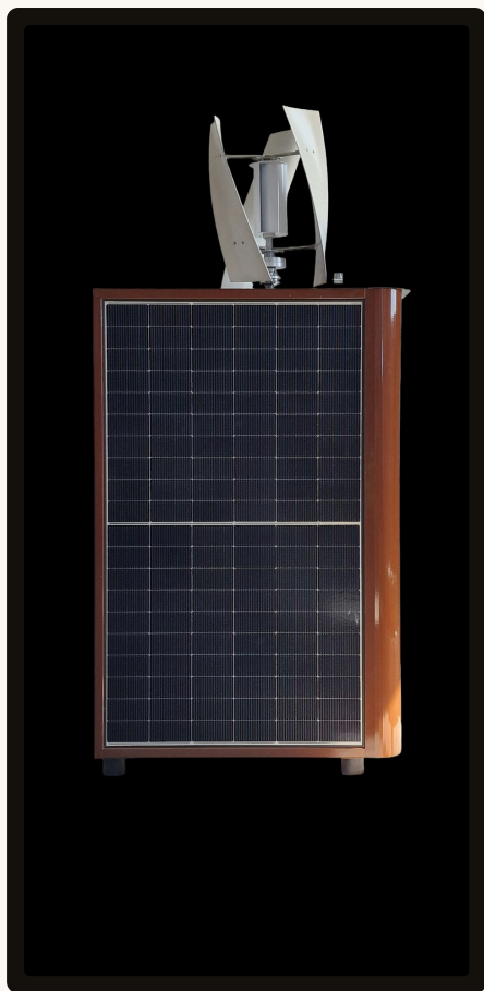
Parte trasera — 2 paneles bifaciales y aerogenerador vertical
