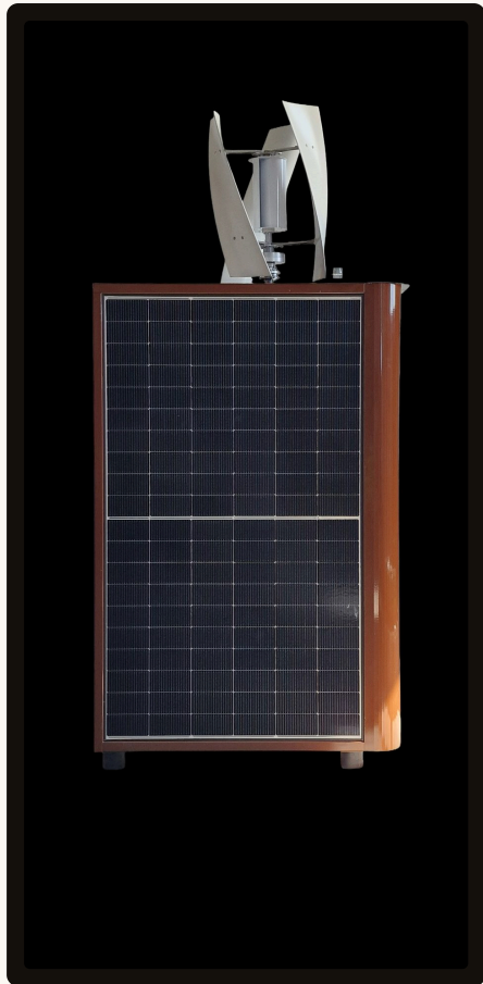
Rückseite — 2 bifaziale Module und vertikales Windrad
